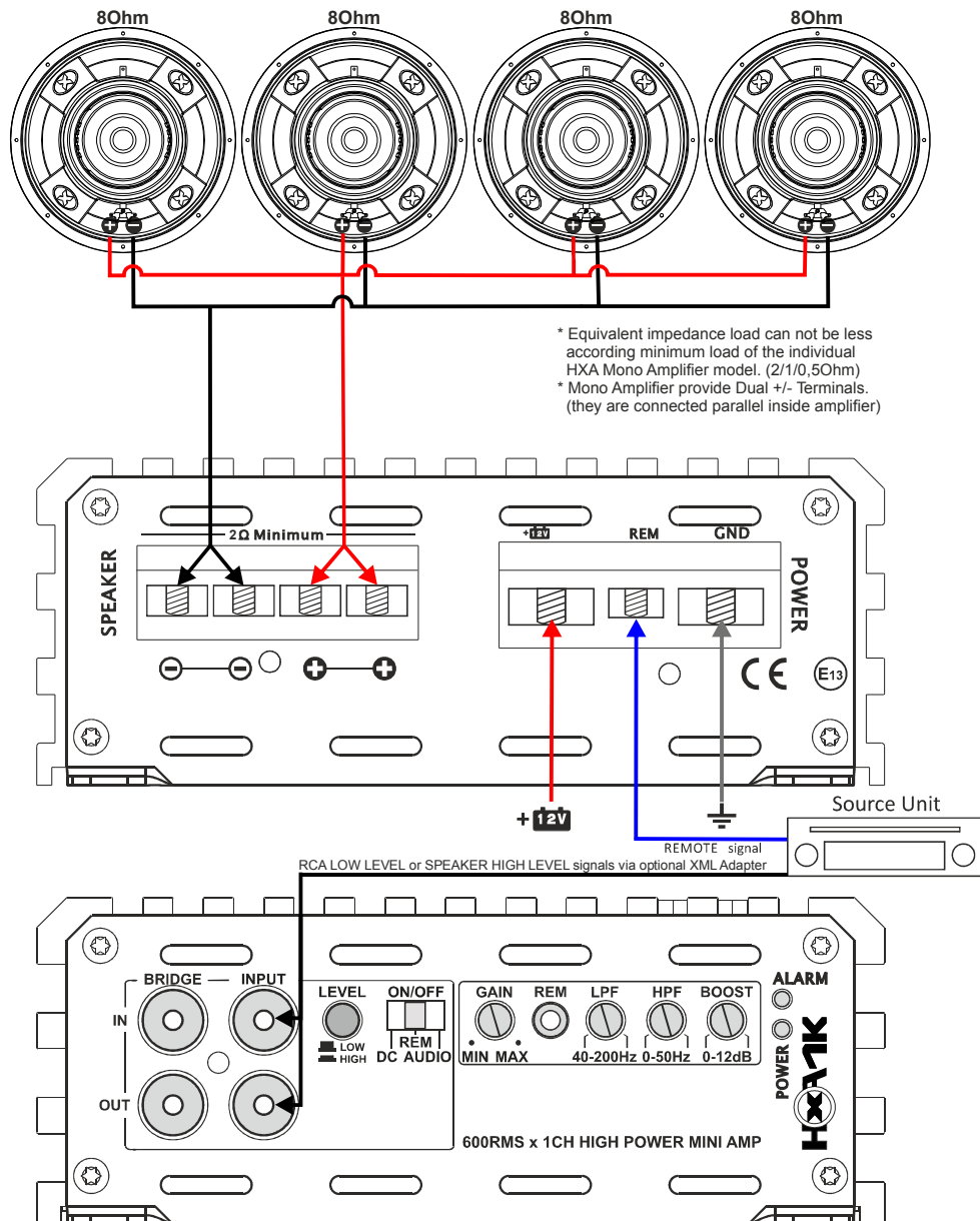
Fig 5. HXA 1K / HXA 2K / HXA 3K / HXA 4K / HXA 5K wiring (1 Channel Mode)
